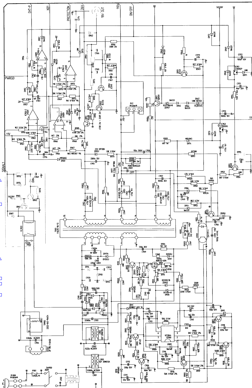
POWER AND DEFLECTION CIRCUIT DIAGRAM CL2156TAN SCHÉMA DE MONTAGE DE CIRCUIT DE PUISSANCE ET DE DÉVIATION CL2156TAN SCHALTBILD NETZSPANNUNG UND ABLENKUNG CL2156TAN
