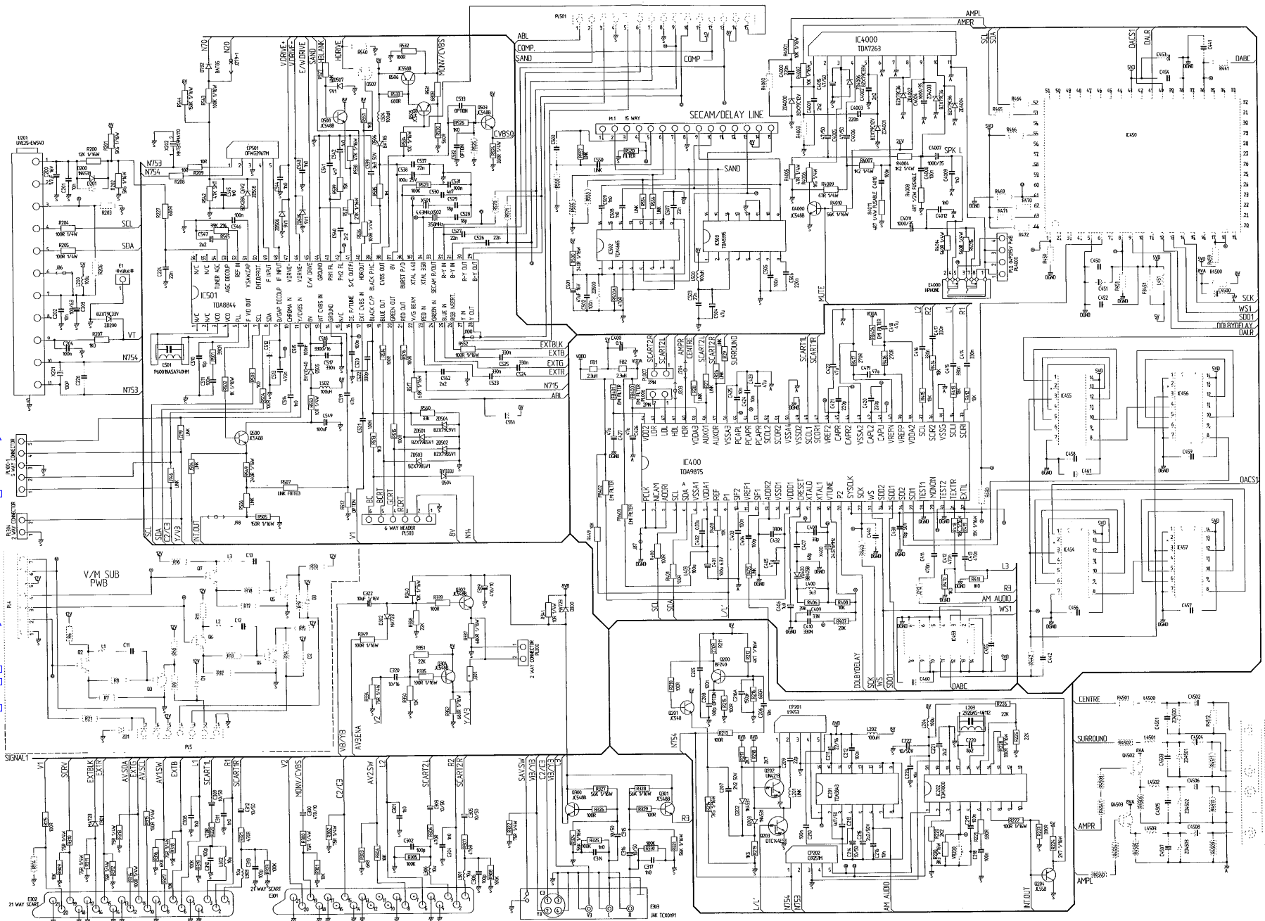
SIGNAL CIRCUIT DIAGRAM CL2856TAN SCHÉMA DE MONTAGE DE CIRCUIT DE TRAITEMENT DU SIGNAL CL2856TAN SIGNALSCHALTBIID CL2856TAN
