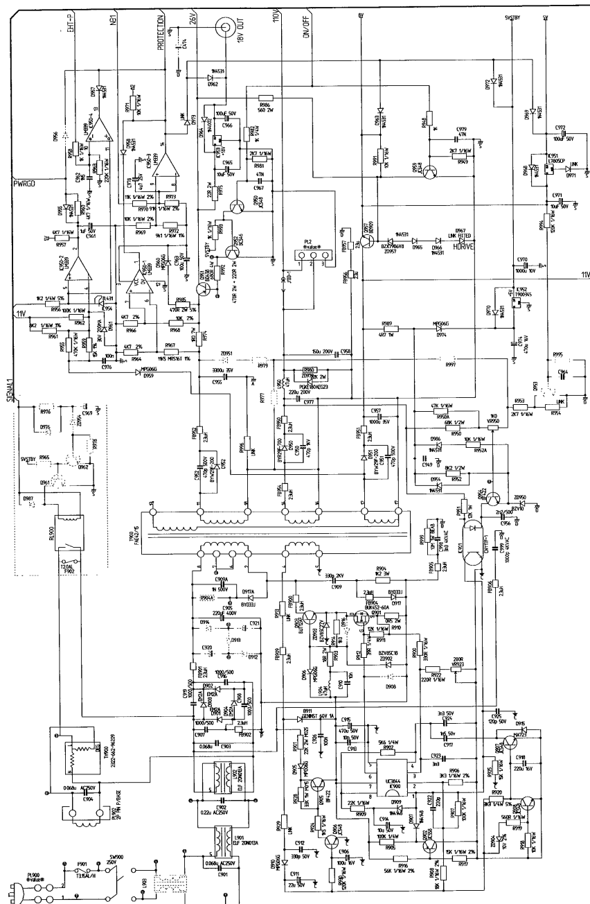
POWER AND DEFLECTION CIRCUIT DIAGRAM CL24W1TAN SCHÉMA DE MONTAGE DE CIRCUIT DE PUISSANCE ET DE DÉVIATION CL24W1TAN SCHALTBILD NETZSPANNUNG UND ABLENKUNG CL24W1TAN
