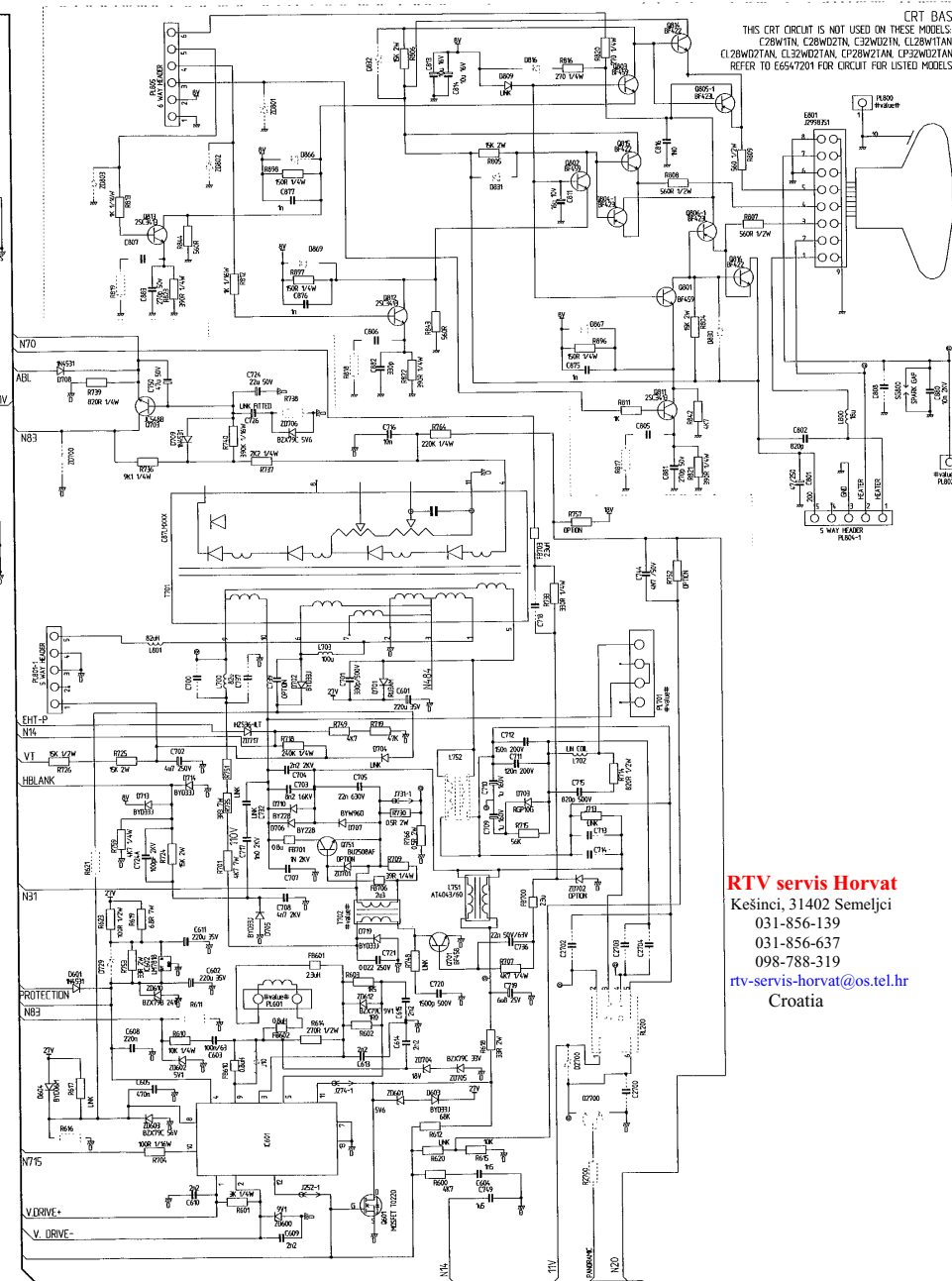
POWER AND DEFLECTION CIRCUIT DIAGRAM CL2886TAN SCHEMA DE MONTAGE DE CIRCUIT DE PUISSANCE ET DE DÉVIATION CL2886TAN SCHALTBILD NETZSPANNUNG UND ABLENKUNG CL2886TAN
