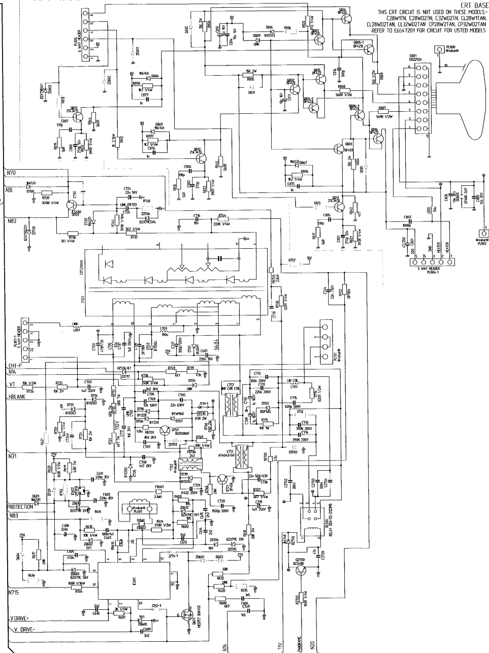
POWER AND DEFLECTION CIRCUIT DIAGRAM CL28WD2TAN SCHÉMA DE MONTAGE DE CIRCUIT DE PUISSANCE ET DE DÉVIATION CL28WD2TAN SCHALTBILD NETZSPANNUNG UND ABLENKUNG CL28WD2TAN
